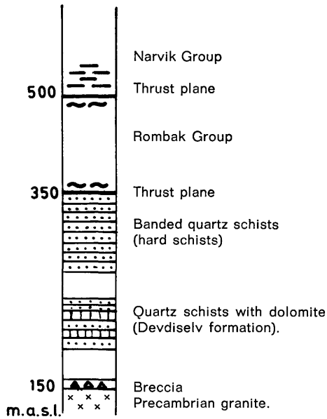
Fig. 17. Schematized profile in the Storffjell Group. Storffjell, Målselv. Skjematisert profil i Storffjell-gruppen, Storffjell, Målselv.
