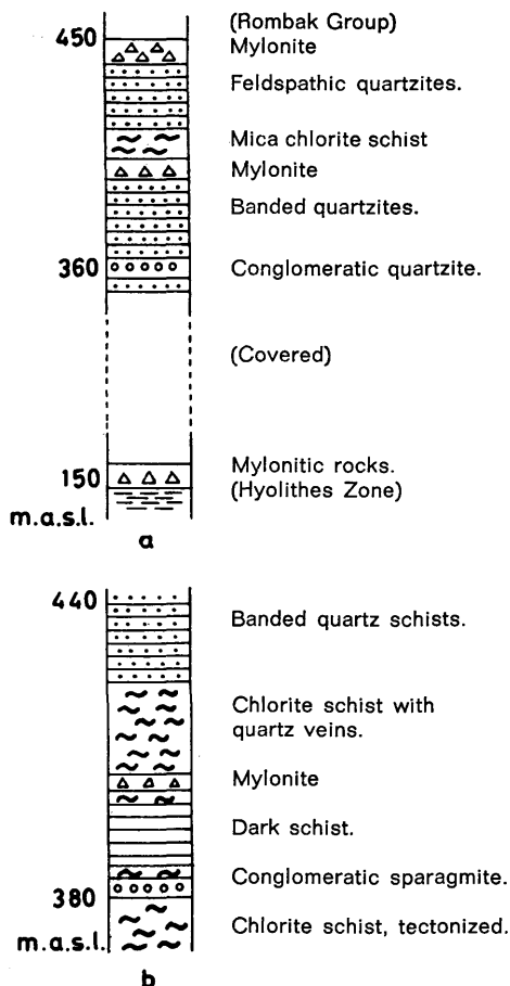
Fig. 19. Schematized profiles in the conglomerate-bearing sequences of the Storffjell Group. (a) W. of Høgskarbus, Dividalen. (b) 5 km S. of Sørmo, Bardu. Skjematiserte profiler i de konglomeratførende deler av Storffjellgruppen.
