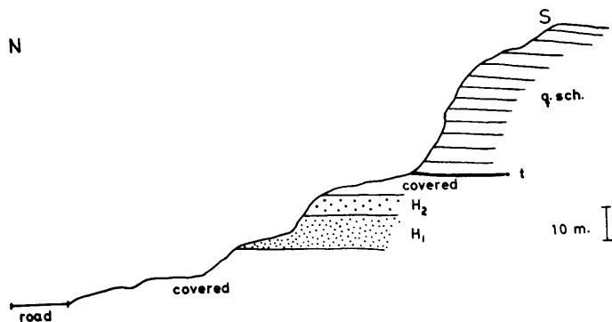
Fig. 16. Hyalolithes Zone ( H_1 and H_2 ) and Storfjell Group. W. of Skjold. Hyalolithes-sonen og Storfjell-gruppen vest for Skjold.
