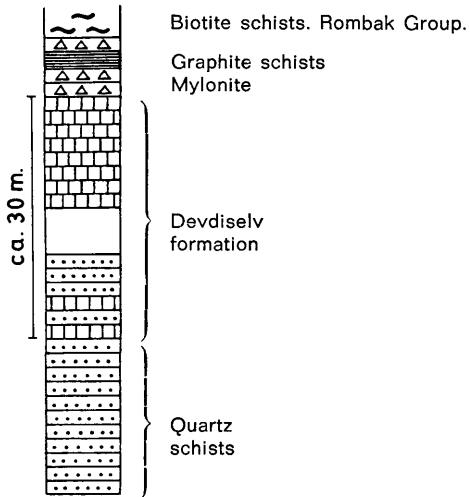
Fig. 18. Schematized profile in the Storffjell Group, Devdiselv, Dividalen. Skjematisert profil i Storffjell-gruppen, Devdiselv, Dividalen.
