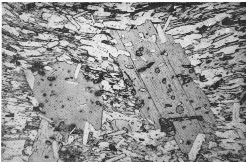
Fig. 35. Porphyroblastic mica schist from the lower part of the Narvik Group, Soløyheia, Lavangen. The biotite porphyroblasts are partly growing across the pre-existing planar structure (orientation of muscovite, biotite, epidote and quartz aggregates) (35x.) Porfyroblastisk glimmerskifer fra den undre del av Narvikgruppen, Soløyheia, Lavangen. Biotittporfyroblastene vokser delvis på tvers av den eldre planstruktur (orientering av muskovitt, biotitt, epidot og kvartzsaggater) (35x).
