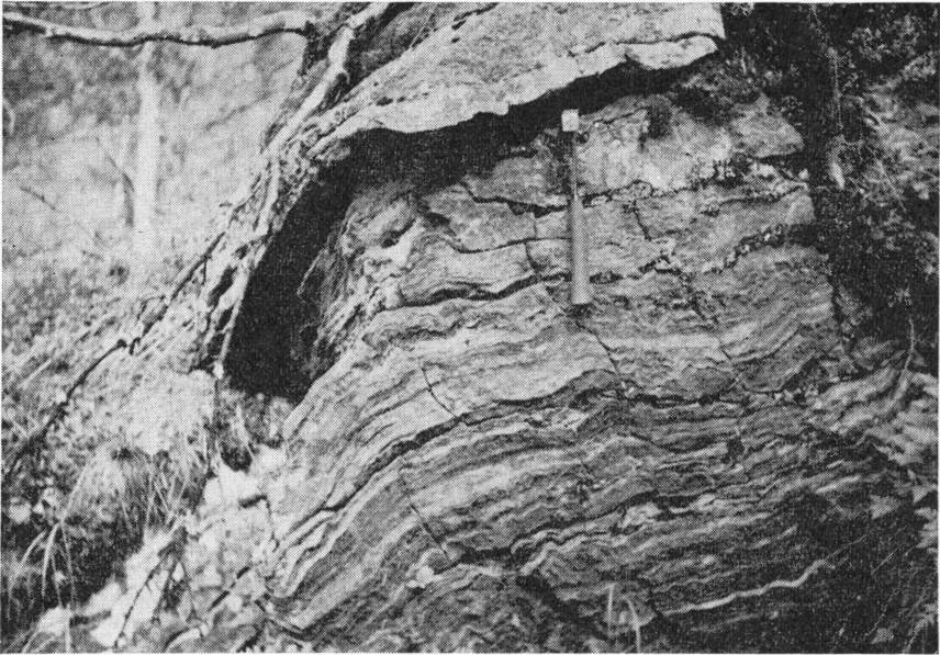
Fig. 22. Banded mica schist in the upper part of the Rombak Group. Rombak profile. Båndet glimmerskifer i den øvre del av Rombakgruppen. Rombak-profilet.
