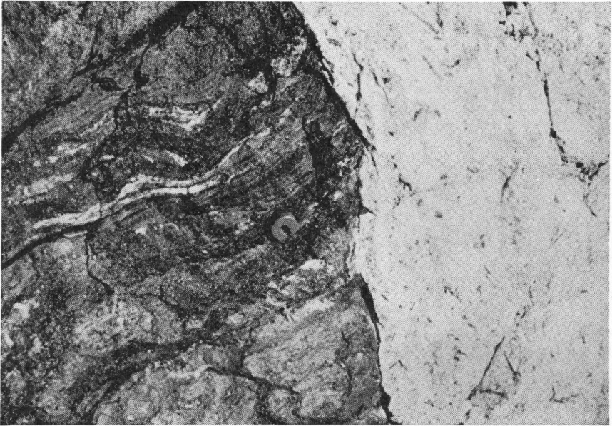
Fig. 30. Banded iron ore cut by granitic dyke, Salangen Group. Storhaugen, Salangen. Båndet jernmalm gjennomsatt av granittgang, Salangen-gruppen. Storhaugen, Salangen.
