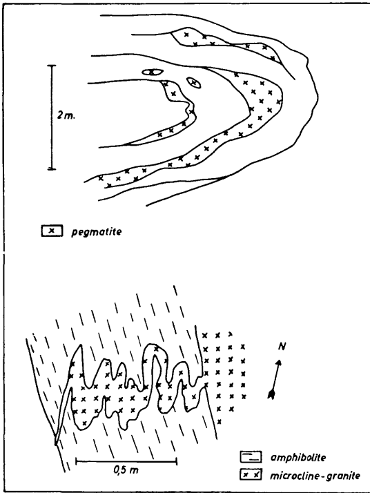
Fig. 12. Pegmatites in the southerly part of the western zone of granitic rocks. For explanation see text. Pegmatitter i den sydlige del av det vestlige granittområde.
