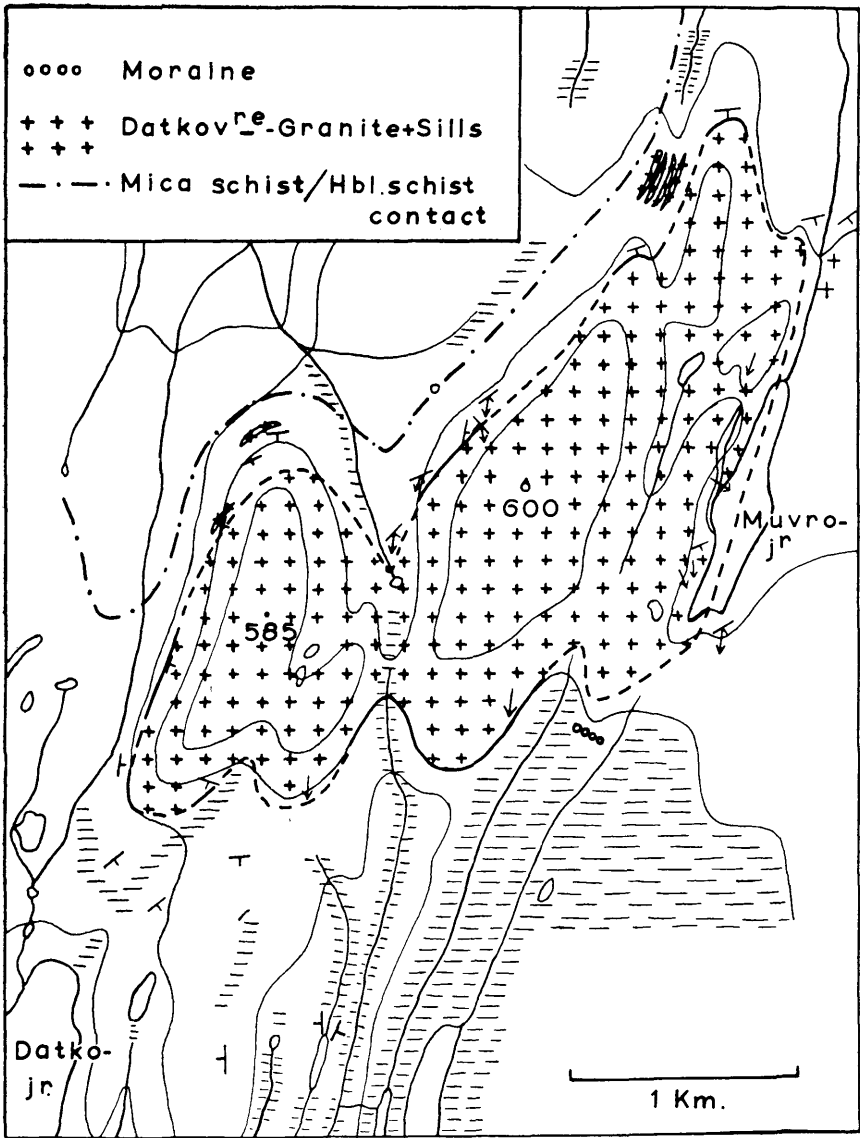
Fig. 10. The Datkovarve granite (after G. C. McCandless). Datkovarve-granitten (etter G. C. McCandless).
