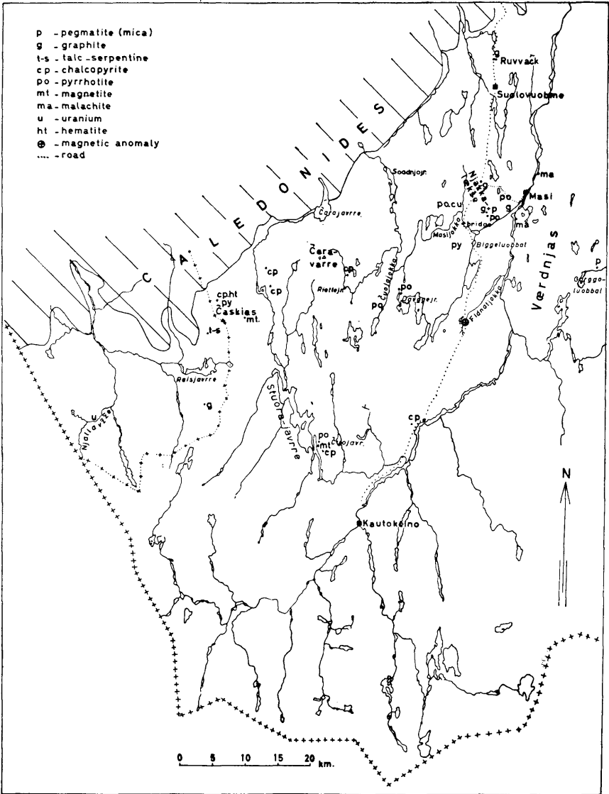
Fig. 21. Map showing location of minerals and rocks of economic interest. Kart som viser opptreden av mineraler og bergarter av økonomisk interesse.
