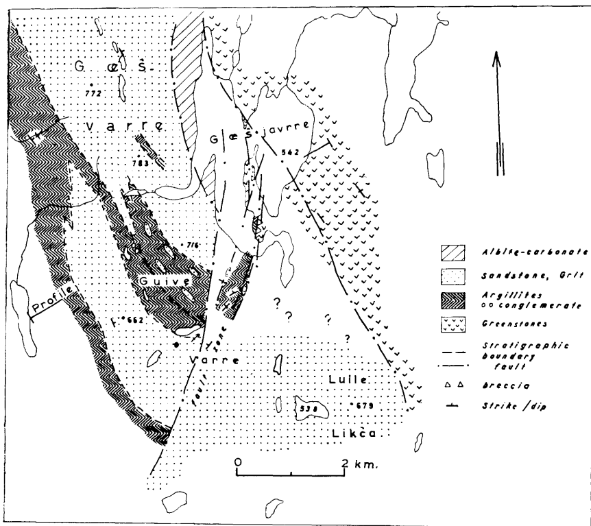
Fig. 3. Geological map of the Gæšvarre—Guivevarre region. For profile see fig. 2. Geologisk kart over området Gæšvarre—Guivevarre. Profil se fig. 2.
