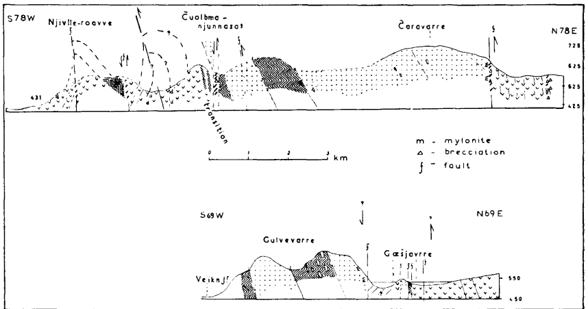
Fig. 2. Profiles across the Čaravarre—Guivevarre ridge. For legend see fig. 3. Tverrprofiler over fjellrekken Čaravarre—Guivevarre. Tegnforklaring se fig. 3.
