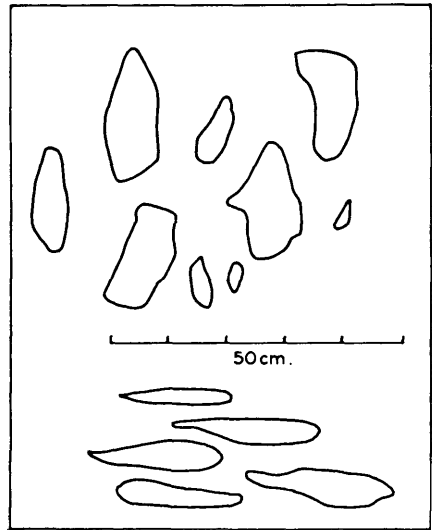
Fig. 5. Drawing of pebbles in the Kautokeino conglomerate: uppermost, on bedding surfaces, lowermost, in section at right angle to schistosity. Tegninger av boller i Kautokeino-konglomeratet: øverst på lagflater, nederst i snitt loddrett på skifriheten.
