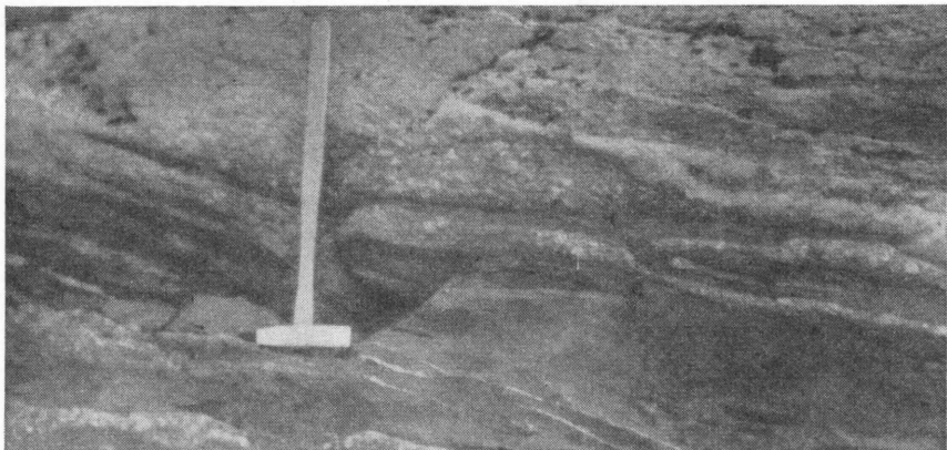
Fig. 2. Benk av grovkornet Børgefjell-granitt med uskarp grense til underliggende skifer. Diffust begrensede slirer med feltspat i nærheten av grensen. Skar syd for fjell 1326 (7.5, 23). Fot. FOSLIE 30/7—30.
