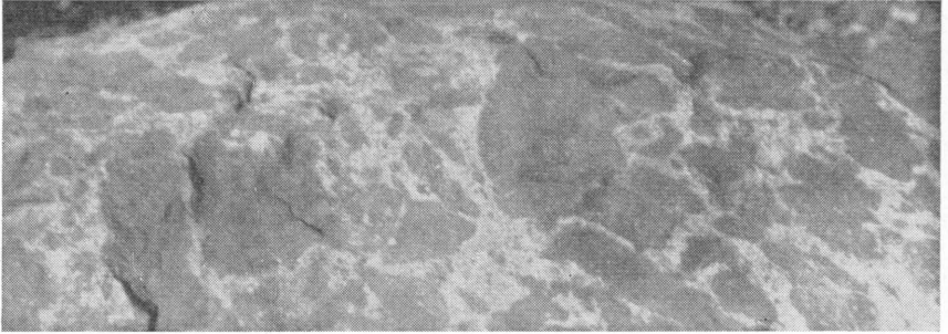
Fig. 13. Gabbro gjennomvevet av trondhjemitt. Linse i glimmergneiss like ved skyveplanet. Store Kjukkelen (8.8, 59). Fot. FOSLIE 17/9—30.
