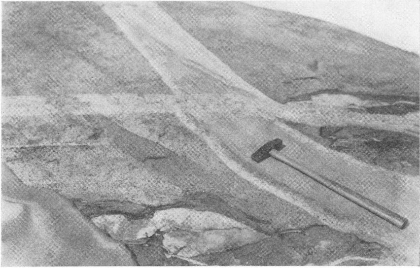
Fig. 18. Granodioritt gjennomslutt av hvit aplitt og pegmatitt (se fig. 19). Øst for toppen av Bleikarfjell (7, 49). Fot. FOSLIE 14/7—31.
