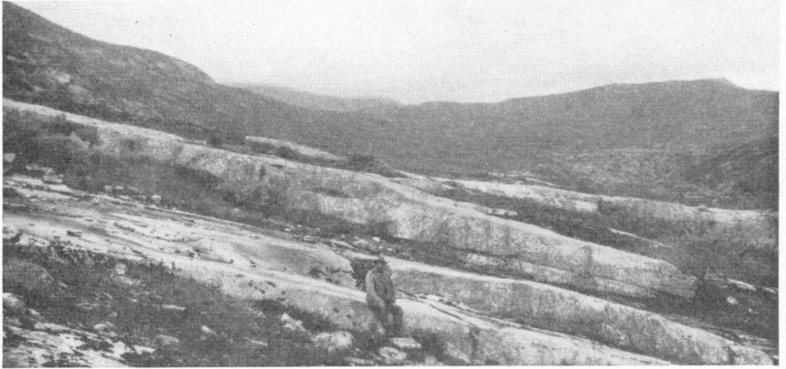
Fig. 14. Kvartsitt. Orrekdalen (8.5, 54). Fot. FOSLIE 22/9—30.
