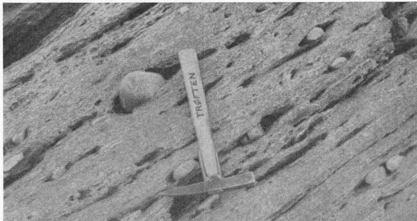
Fig. 7. Konglomerat med kalksandsteinsgrunnmasse i Liming-avdelingen. Halvmilstangen, Limingen (52, 46). Fot. bergingeniør P. F. TRØFTEN 1954.
