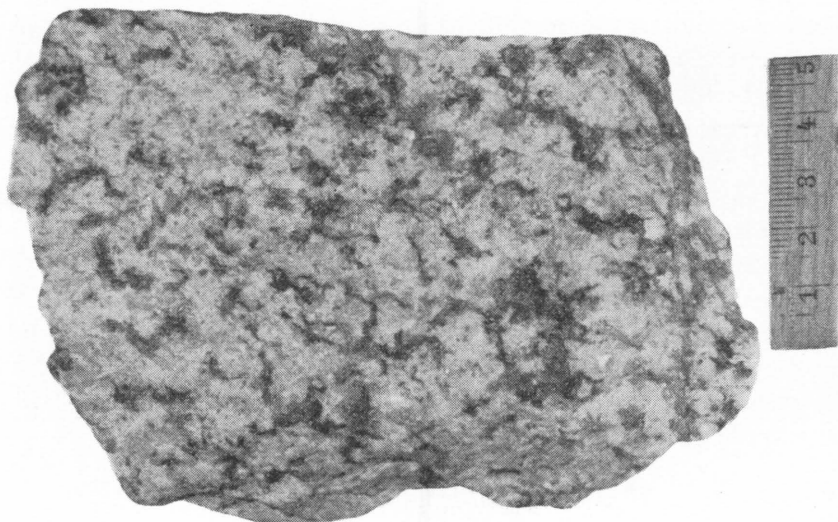
Fig. 1. Granittisk gneis, bekk på nordsiden av Jetnamen jaure (7, 29.2), 57B 302, materiale til analyse 1.
