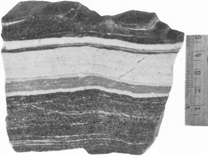
Fig. 11. Båndet grønnstein, ved veien Gjersvik—Brekkvasselv (51.5, 32), 57A 201.
