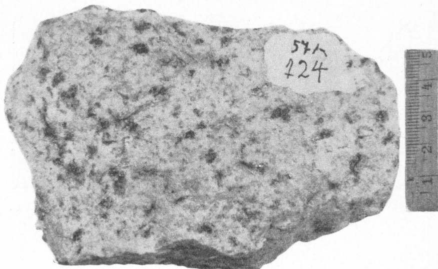
Fig. 17. Granodioritt, tjern øst for høgd 606 (59, 41), 57A 124.
