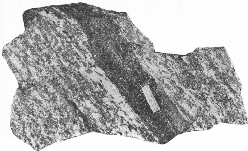
Fig. 4. Båndet amfibolitt, veiskjæring Hurum (9, 55). \times \frac{1}{2} .
