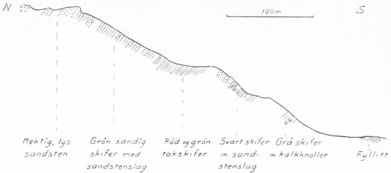
Fig. 6. Profil av Mellsekkavdelingen i sydskråningen av Mellane like vest for østgrensen av kartområdet Slidre.
