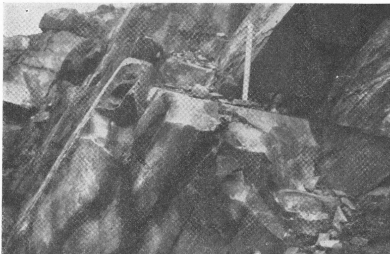
Fig. 3. Glimmerførende grunnfjellskvartsitt ved Beitehaugen (14.5, 52.2), lagene faller bratt mot vest.
