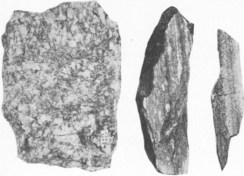
Fig. 10. Syenittmylonitter fra høgd 1143 (19.3, 55.4) øst for Raudfjorden. I stykket til venstre er det rikelig med store feltspatkorn (mikroklin), stykkene til høyre viser hvordan disse etter hvert males opp og forsvinner. Syenite mylonites from hillock 1143 (19.3, 55.4), showing progressive trituration of the microcline porphyroclasts.
