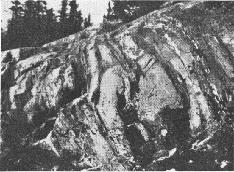
Fig. 7. Mørk skifer med kvartsittlag (lyse på forvitret overflate), lagene faller mot nordøst, Mellsennavdelingen, Mellbyhøgda (11.3, 46.5).
