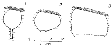
Fig. 20. Profiler fra Grønligrøtten (se kart fig. 19) 1. Fiskekroken. 2. Nord- vestgangen (se kart fig. 19 og pl. 15, 2). 3. Storkirken.
