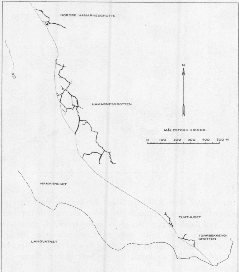
Fig. 12. Hamarnesgrotten og huler i nærheten.
