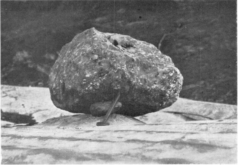
Fig. 1. Pikhaugene. Blokk av porfyrgranitt, etterlatt av isen på kalkfjell. Ved oppløsning er dette tæret ned, så blokken nå hviler på en pillar ca. 10 cm høy. Se også Pl. 8, fig. 2. G. H. 1/8 1937.
