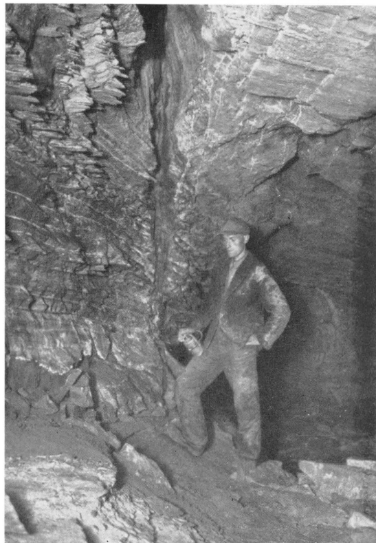
Fig. 2. Hamarnesgrotten. Foto. sta. 1 på kart fig. 7. Nord-sør takspalte. Strekningstruktur vest-øst sees i taket. G. H. 18/8 1936.
