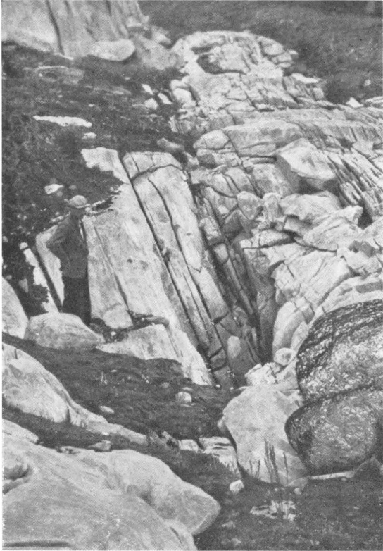
Fig. 1. Inngang til Pikhauggrotte nr. 1. Kart fig. 18. Ser mot nordøst. Se også Pl. 7, fig. 2. G. H. 1/8 1937.
