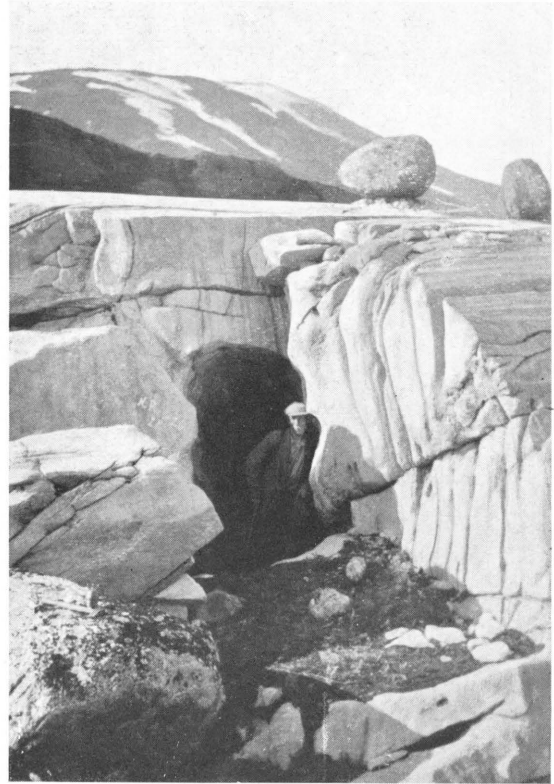
Fig. 2. Inngang til Pikhauggrotte nr. 2. Kart fig. 18. Ser mot nord. Over inngang sees porfyrblokk på pillar. Se også Pl. 6, fig. 1. G. H. 13/8 1934.
