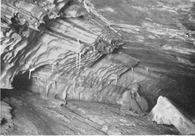
Fig. 1. Olavsgrotten. Vest for „bjørnehiet“ (kart fig. 27). Hule med rektangulært tverrsnitt. Opplosningsskåler og tynne dryppstein. Tak og bunn er også kalk. G. H. 26/8 1935.
