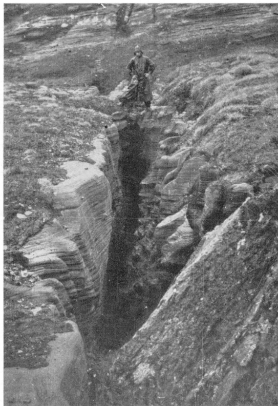
Fig. 2. Glomfjorden. Navnløsvatn. Sprekk på platå øst for Grotte nr. 2. Kart fig. 32. G. H. 18/9 1939.
