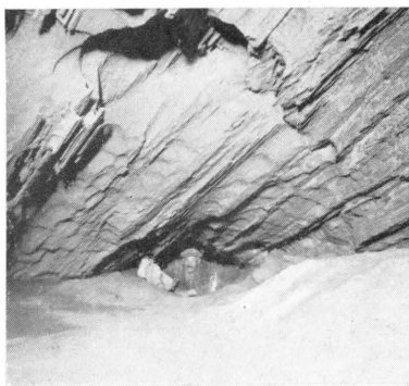
Fig. 1. Hamarnesgrotten. Foto. sta. 2 (kart fig. 8). „Trangen“ med avleiringer av sand. G. H. 31/8 1934.
