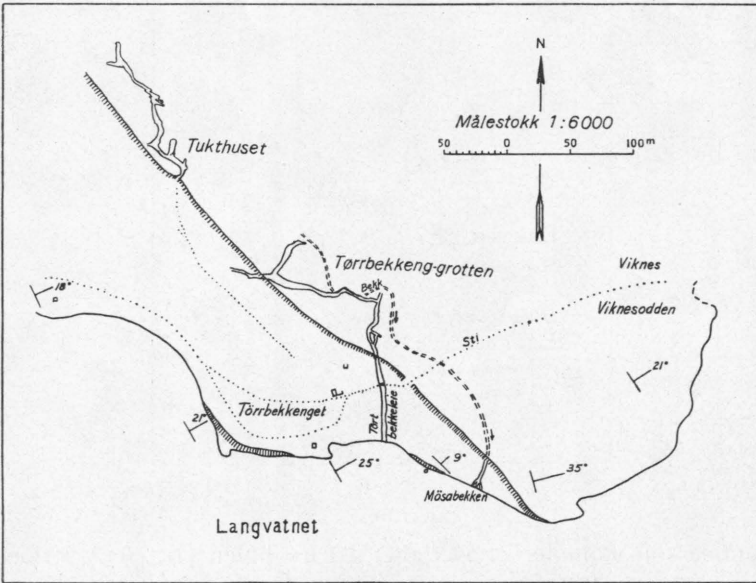
Fig. 4. Strøket omkring Tørrbekkenget ved Langvatnet.
