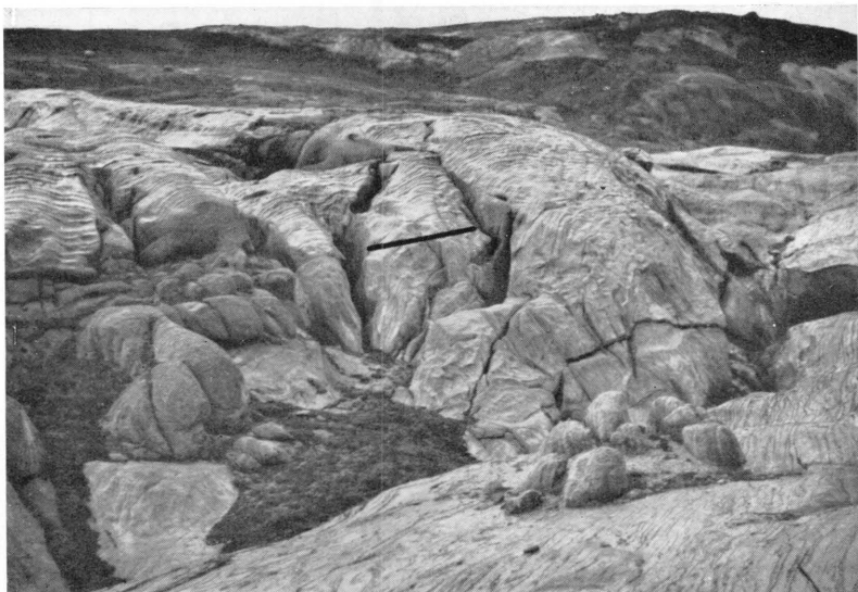
Fig. 1. Glomfjorden. Sørøst for 640 m-høyden nord for Storglomvatnet (kart 1:100 000). Kalkfjell med karren. Strek er 1,5 m. G. H. 27/8 1936.
