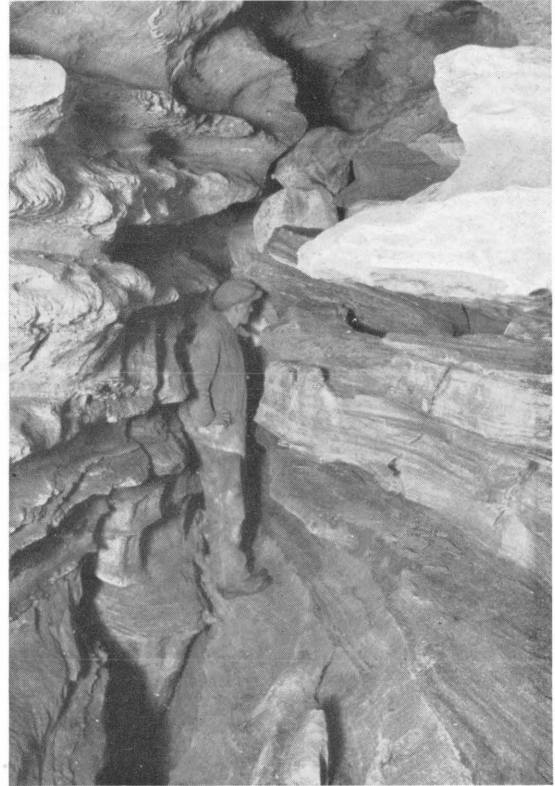
Fig. 2. Stokkvikgrotten. Litt lengre inn enn foregående bilde. Sammenlign profil fig. 3. G. H. 12/9 1939.
