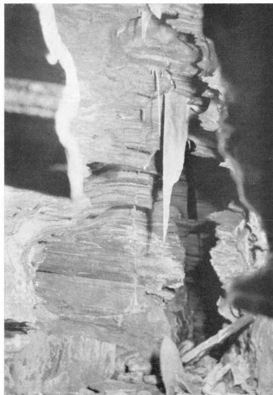
Fig. 2. Larshullet. Dryppstein på sprekke 10 m v. for Fossehallen, kart fig. 24. Stalagmitt 71 cm lang. På liggen tilsv. stalaktitt. Mørke „plater“ t. v., og t. h. er granitt injisert i kalken og med strekningstruktur i ø-v. retn. (= hulens lgd.-retn.). G. H. 22/s 1934.
