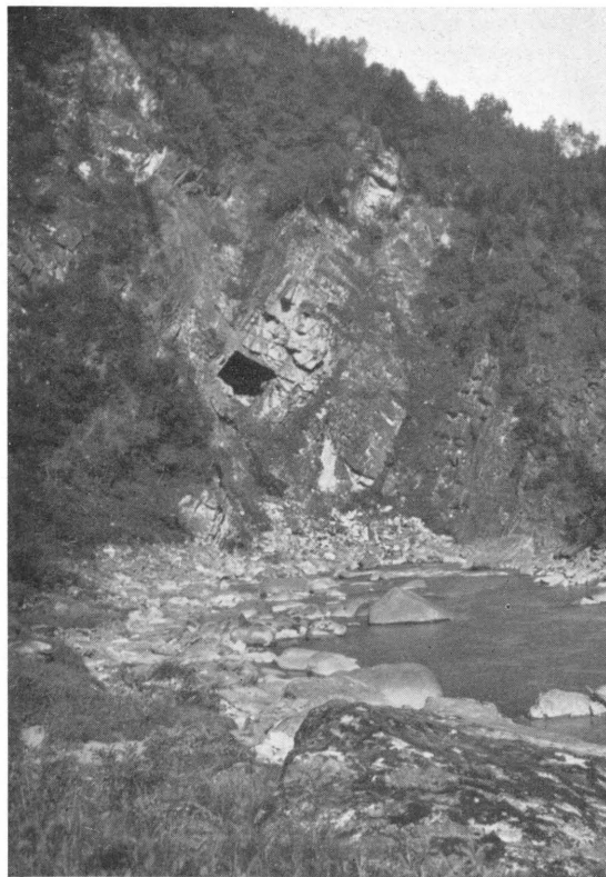
Fig. 2. Bredekhulen. Nedre dagåpning, ca. 6 m høy. I forgrunnen Stormdalsåga. G. H. 4/9 1939.
