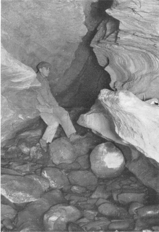
Fig. 1. Stokkvikgrotten. Hule dannet etter øst-vest-gående sprekk. Nær åpningen og sett mot denne (vestover). G. H. 12/9 1939.
