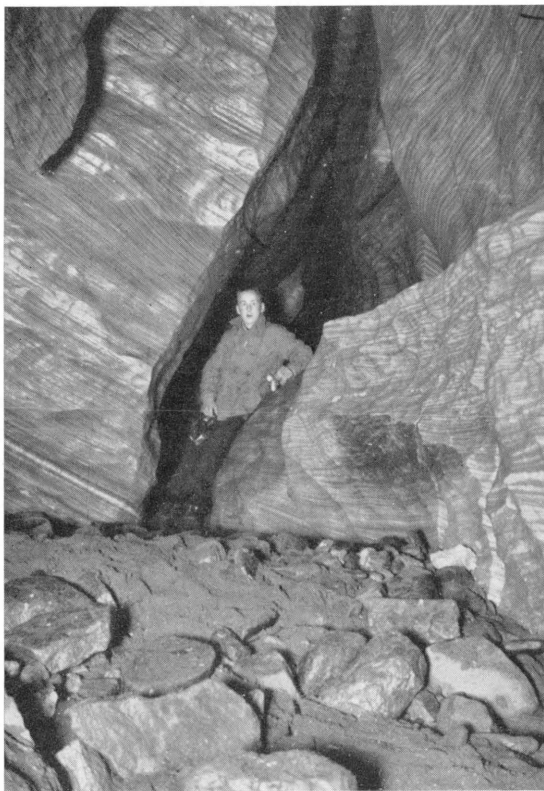
Fig. 1. Glomfjorden. Navnløsvatn. Grotte nr. 2. Nord-sør sprekk nær hulens bunn, ser mot nord. Kart fig. 32. G. H. 18/9 1939.
