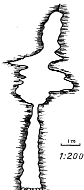
Fig. 3. Stokkvikgrotten. Ser mot grottens utgang (retning ca. N 85° W). Se også pl. 2, fig. 2.
