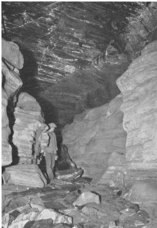
Fig. 1. Setergrotten. Foto. sta. ca. 30 m sør for Prekestolen (kart fig. 21). Ser mot nord. Glimmerskifer i taket. G. H. 1/9 1939.
