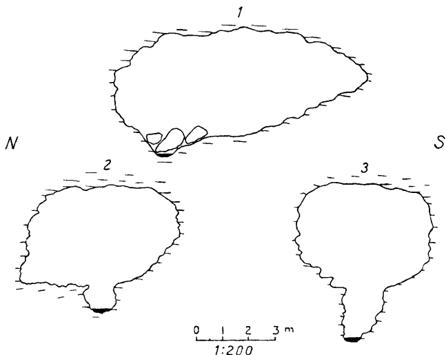
Fig. 26. Profiler fra Larshullet
