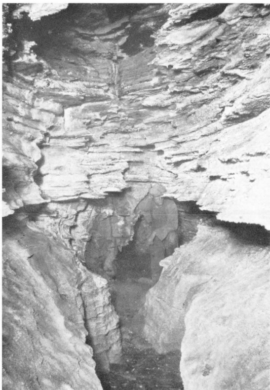
Fig. 1. Reingardsligrotten. Foto. sta. 1, kart fig. 29. Hulen følger øst-vestgående spalte. Fremspringende kanter av tungt oppløselige mineraler (glimmer etc.). Se også Pl. 9, fig 2. G. H. 25/s 1935.
