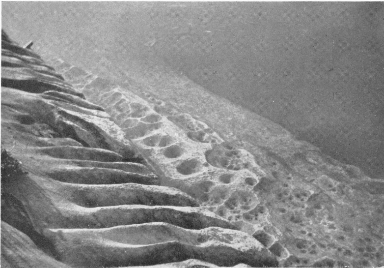
Fig. 2. Reingardslivatnet. Strand ved hus på sørsiden (kart fig. 22). Karren og eiendommelige fordypninger i kalk umiddelbart under vannflaten („solution pits“). G. H. 18/8 1935.
