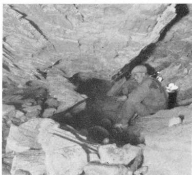
Fig. 2. Larshullet. Foto. sta. ca. 25 m øst for fastmerke 1 (kart fig. 24). Ser østover. Som de andre stereoskopiske bilder er dette tatt med to like kameraer, som for tilfellet er stilt opp med en avstand av ca. 35 cm. Avstand til mann i fig. 2 er ca. 8 m. G. H. 22/8 1934.
