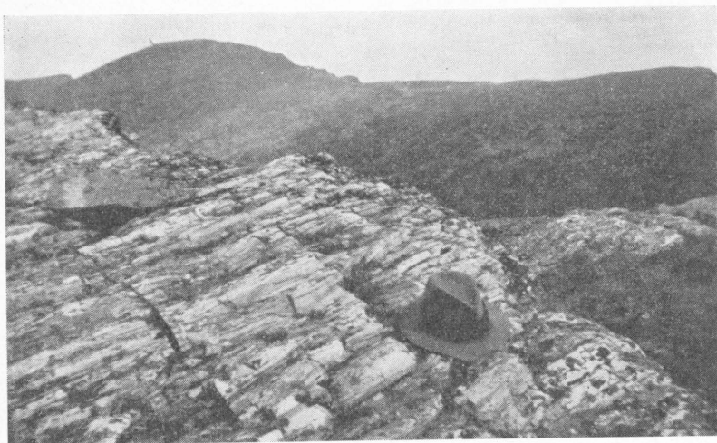
Fig. 12. Kvartskonglomerat med strukne boller i Marsteinshøgda. I bakgrunnen mot øst søndre Langsuen.
