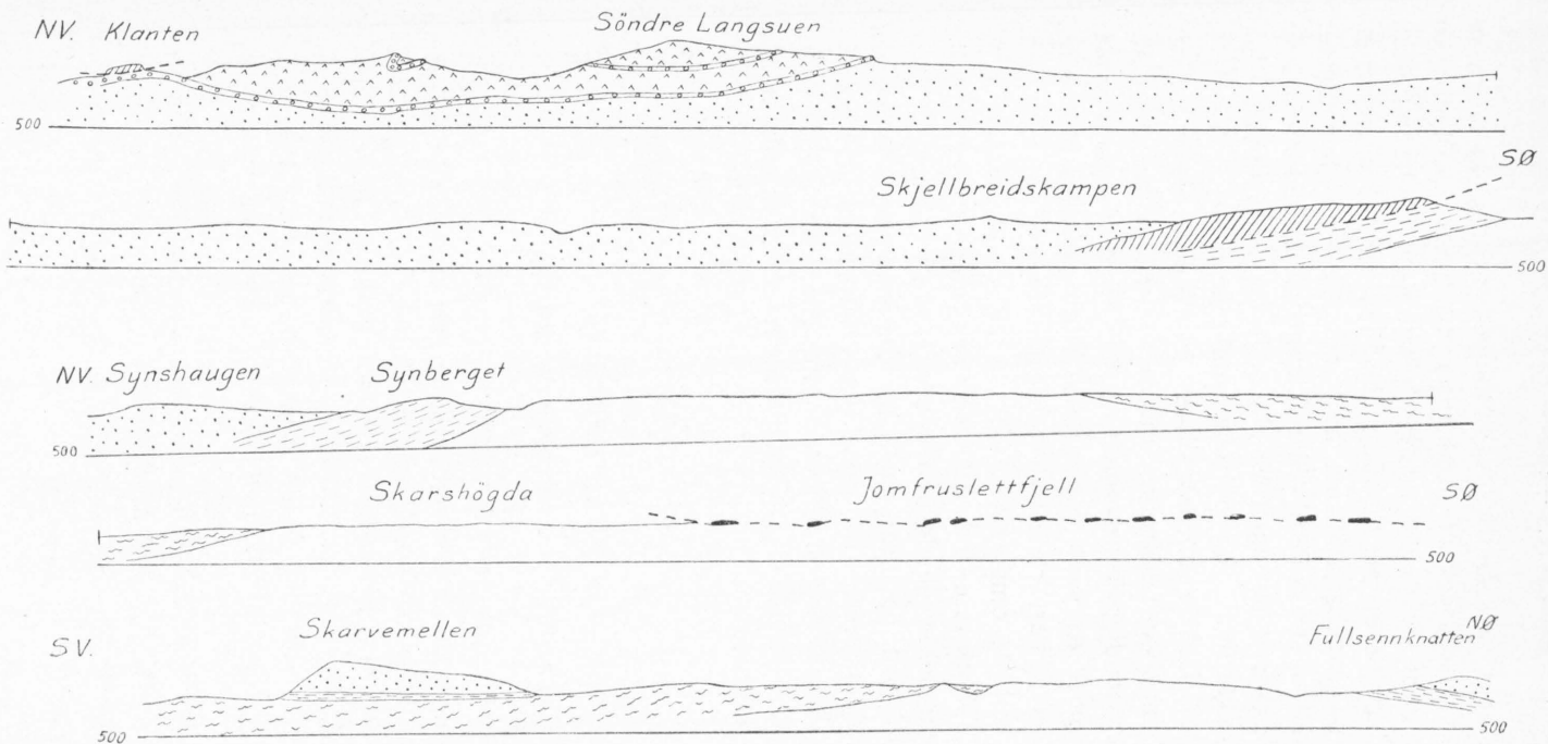
Fig. 2. Profiler over kartområdet Nordre Etnedal. Betegnelser som fig. 1. Målestokk 1:100 000 både for høide og lengde.
