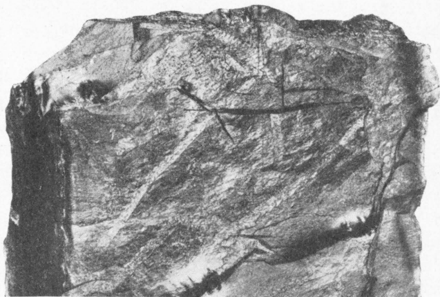
Fig. 4. Fyllitt med graptolitter fra ved bekken syd for Hovsjøen, naturlig størrelse. Øverst en kort og bred Phyllograptus , nedenfor grenstykker av Didymograptus .
