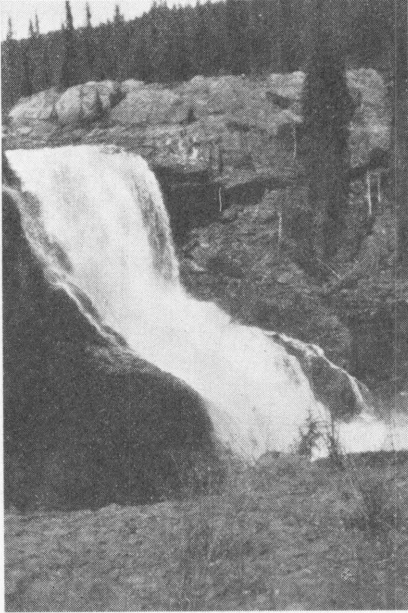
Fig. 7. Høgefoss i Etna. Synnfjellsandsten øverst i styrtningen, under og nedenfor grønn kambrisk skifer. I forgrunnen avfall fra et litet skiferbrudd.
