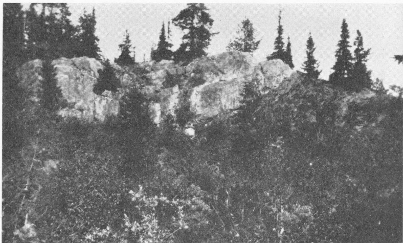
Fig. 6. Synnfjellsandsten og underliggende kambrisk skifer i høiden pkt. 804 i den sydvestligste delen av kartområdet.
