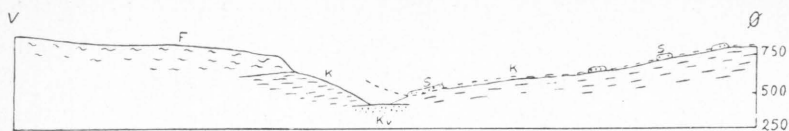
Fig. 10. Profil langs sydgrensen for kartområdene Nordre Etnedal og Slidre. Kv — Kvartssandsten, K — Kambrium, F — Fyllittavdelingen, S — Synnfjellsandsten. Se teksten.
