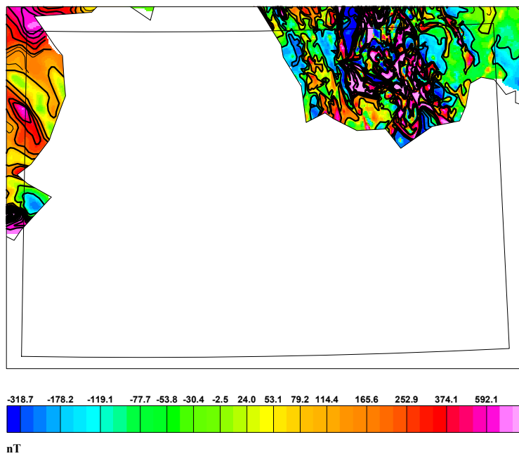
AEROMAGNETISK ANOMALKART Magnetiske feltet referert til ICGF 1965 AEROMAGNETIC ANOMALY MAP Magnetic field referred to ICGF 1965
