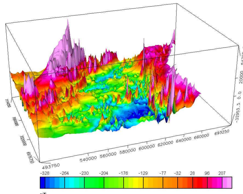
AEROMAGNETISK 3D ANOMALIKART Magnetisk felt referert til IGRF 1965.0
