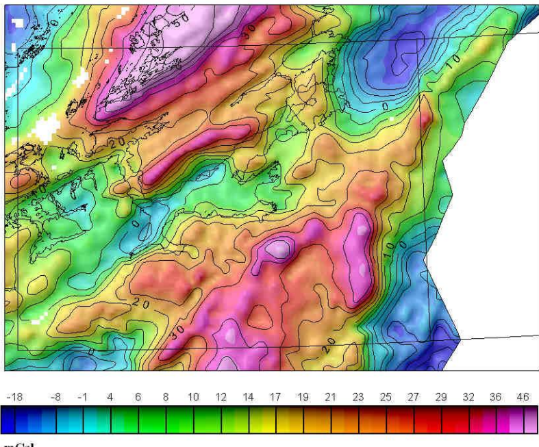
GRAVIMETRISK RESIDUALKART GRAVITET RESIDUAL MAP
