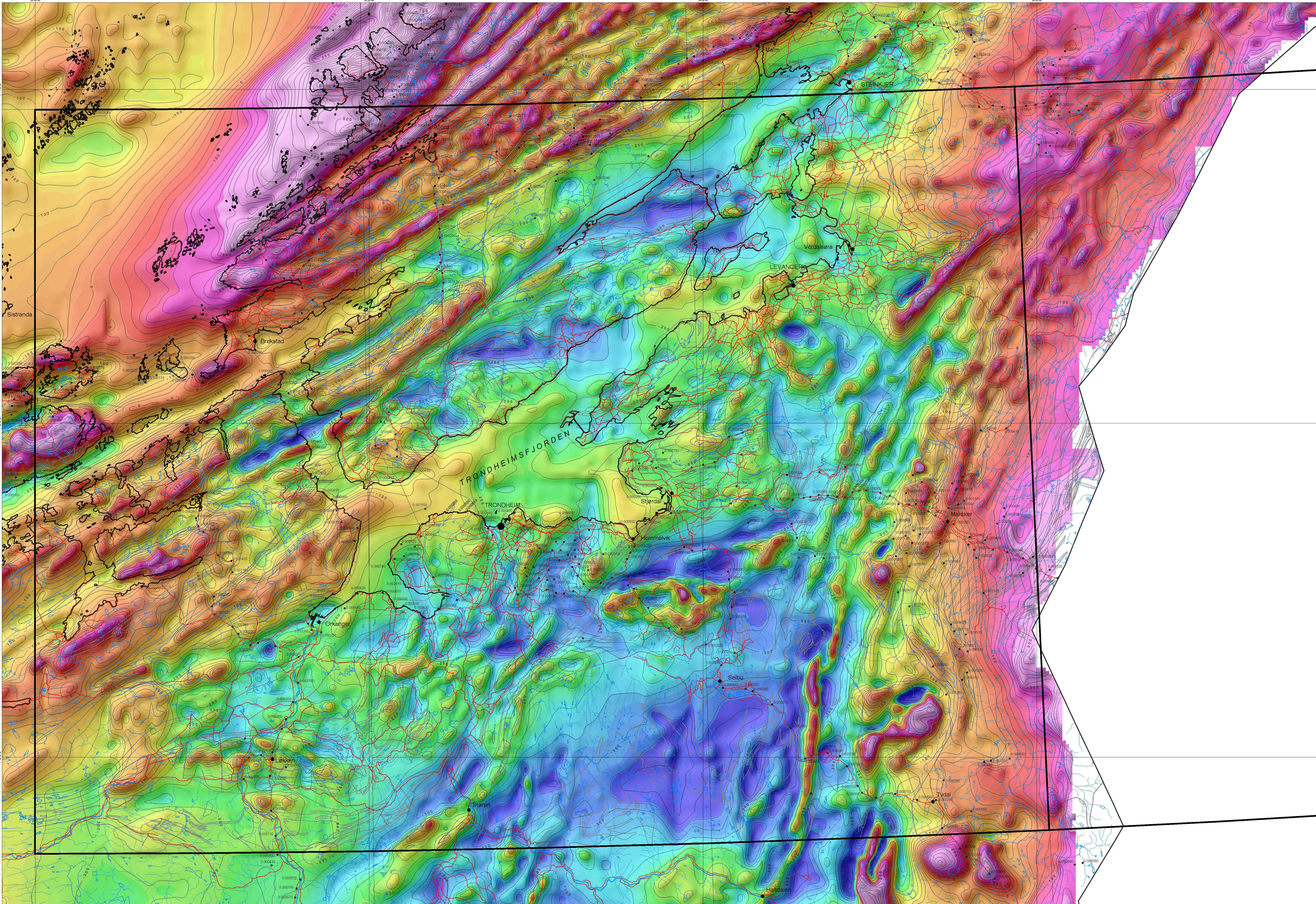
TYNGDEANOMALIKART Tyngdekart til bruk sammen med GRAVITET ANOMALIKART
