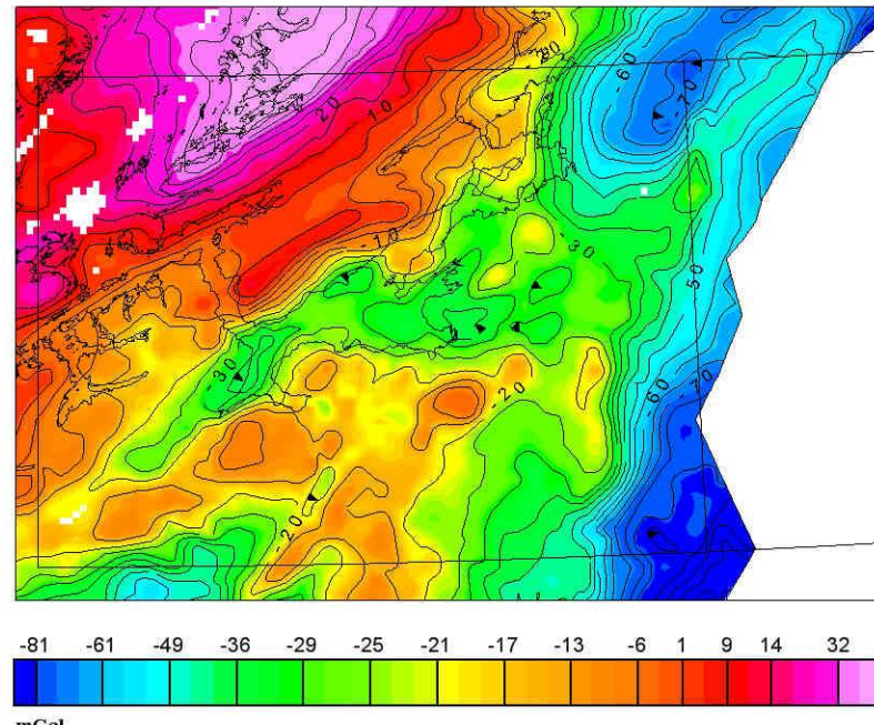
TYNGDEANOMALIKART Tyngdekart til bruk sammen med GRAVITET ANOMALIKART
