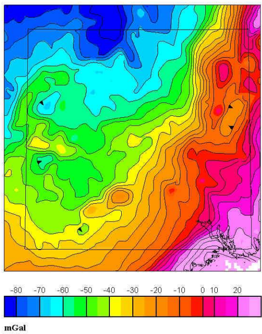
TYNGDEANOMALIKART Terrengkorrigerte bouguer anomalier
