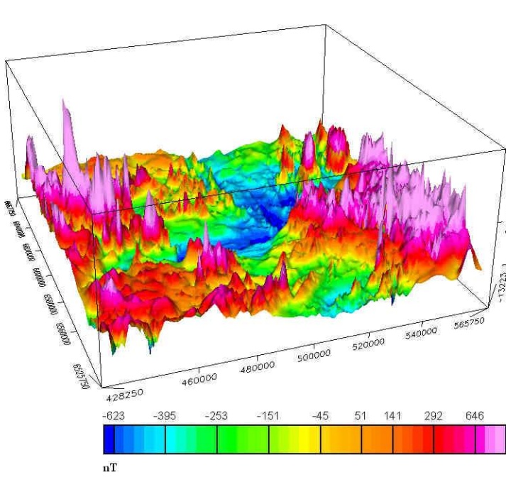
AEROMAGNETISK 3D ANOMALIKART Magnetiske felt referert til DGRF 1965.0
