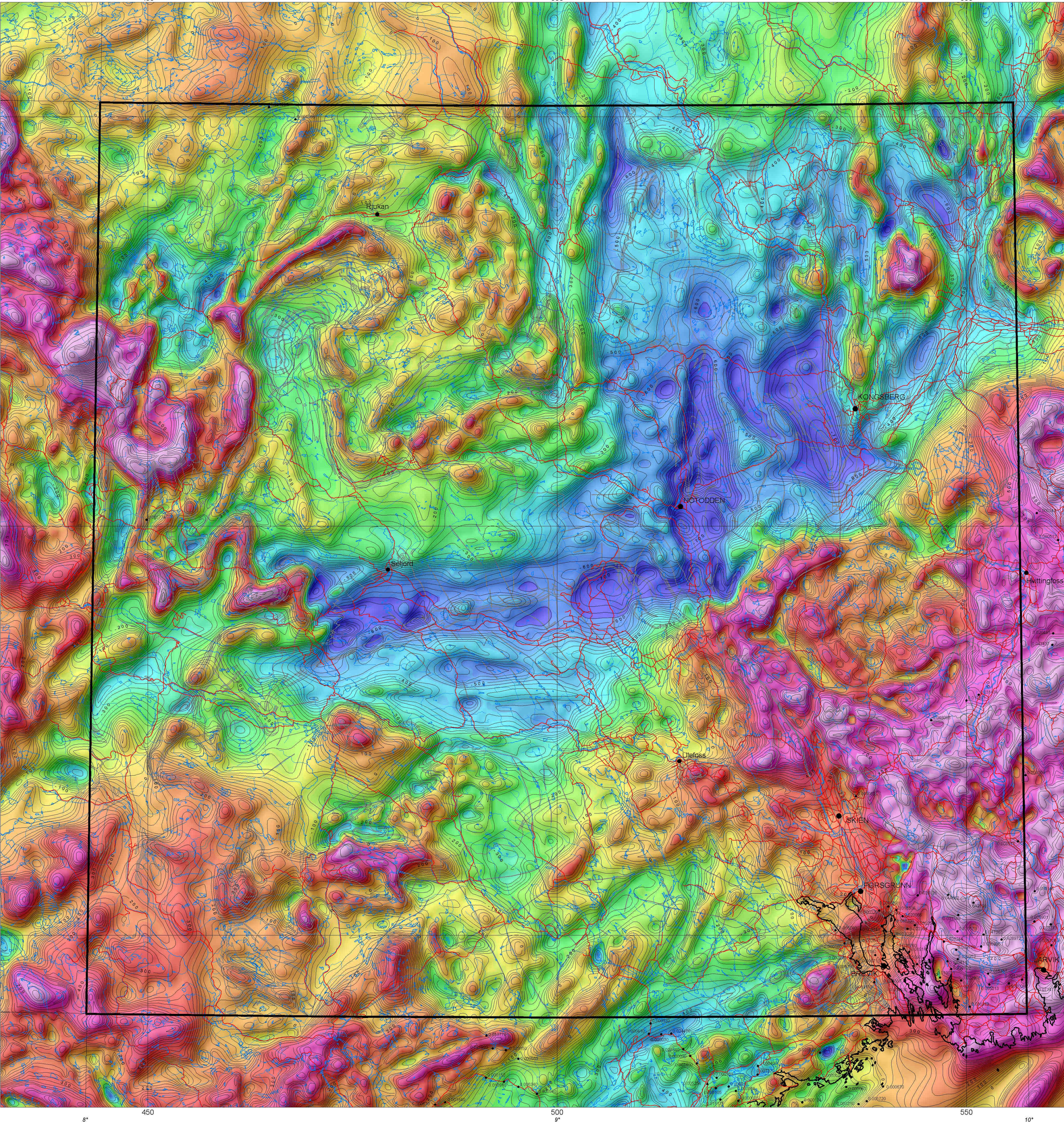
TYNGDEANOMALIKART Terrengkorrigerte bouguer anomalier
