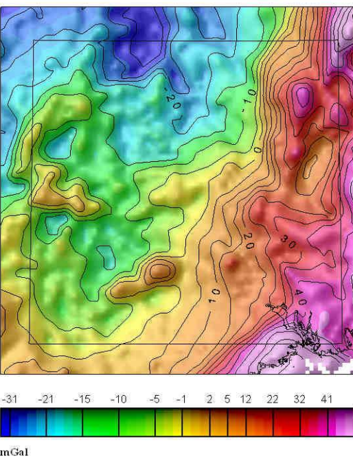
GRAVIMETRISK RESIDUALKART
