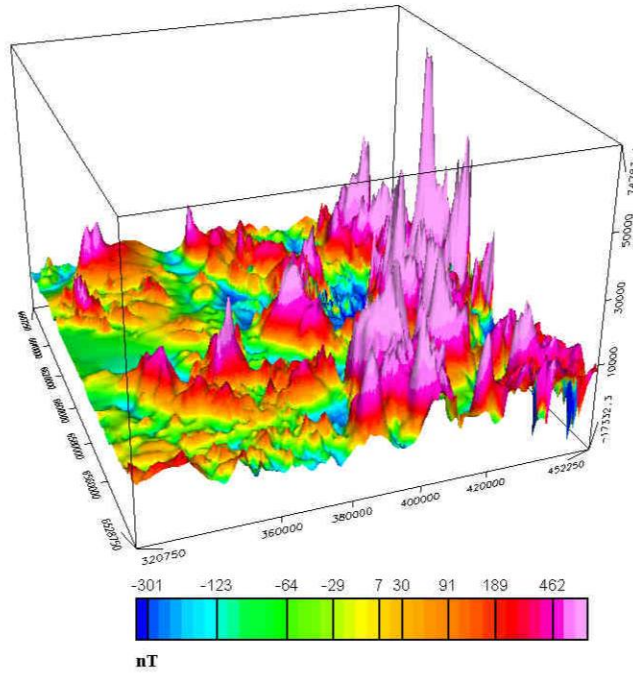
AEROMAGNETISK 3D ANOMALIKART Magnetfeltet referert til DGRF 1965.0 AEROMAGNETIC 3D ANOMALY MAP Magnetic field referred to DGRF 1965.0
