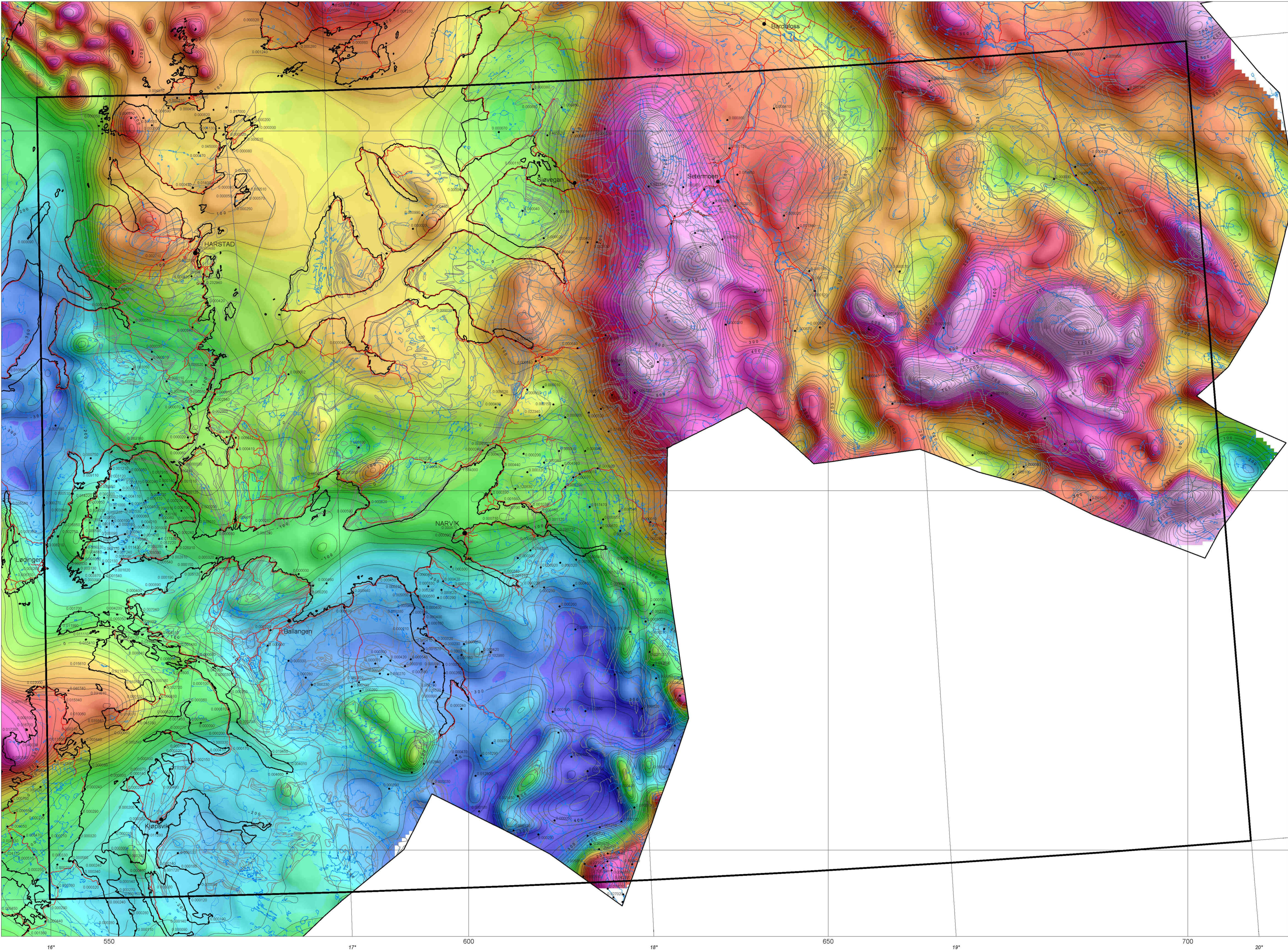
TYNNEANOMALIKART Tynnekorrigerte lugepunkt anomalier GRAVITY ANOMALY MAP Terrain-corrected bouguer anomalies
