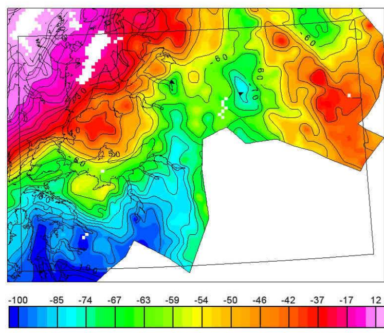
TYNNEANOMALIKART Tynnekorrigerte lugepunkt anomalier GRAVITY ANOMALY MAP Terrain-corrected bouguer anomalies
