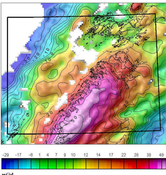
GRAVIMETRISK RESIDUALKART Målestokk referert til DGRF 1965.0 GRAVITY RESIDUAL MAP Magnetic field referred to DGRF 1965.0
