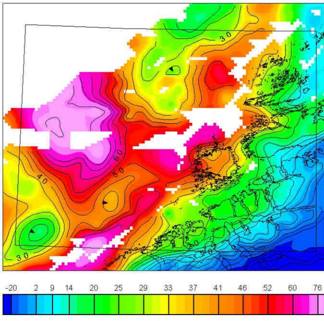
TYNGDEANOMALIKART Terrengkorrigerte høydeanomalier GRAVITY ANOMALY MAP Terrain-corrected height anomalies
