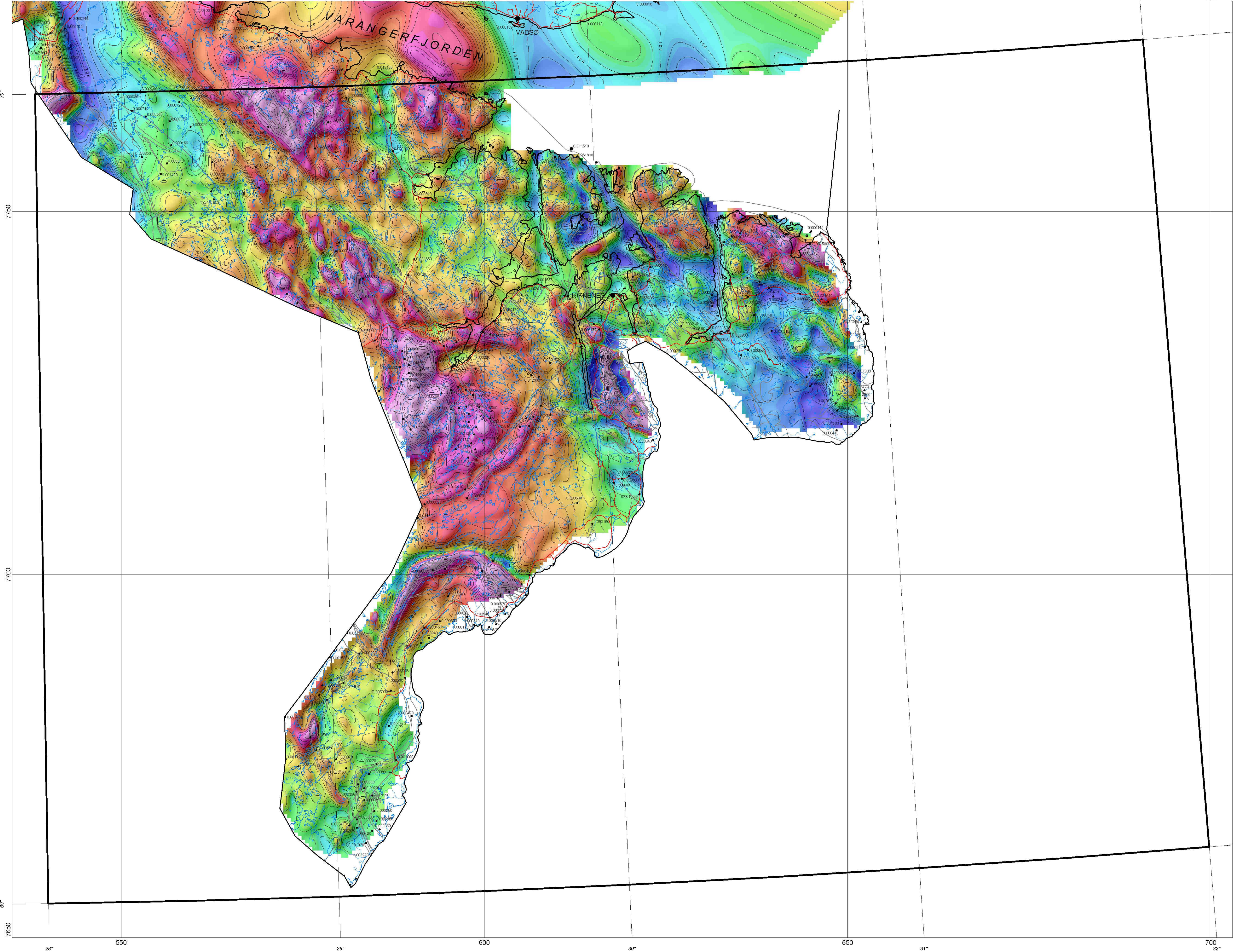
TYNGDEANOMALIKART Terrorgrunnsgeologiske kartserie 1:250 000 Terrain-corrected bouguer anomalies
