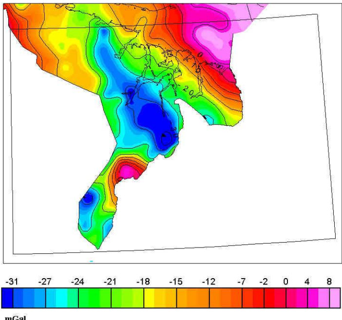
TYNGDEANOMALIKART Terrorgrunnsgeologiske kartserie 1:250 000 Terrain-corrected bouguer anomalies
