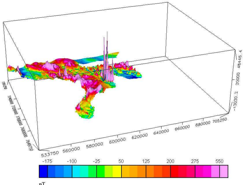
AEROMAGNETISK ANOMALIKART Magnetisk felt referert til DGRF 1965.0 AEROMAGNETIC ANOMALY MAP Magnetic field referred to DGRF 1965.0
