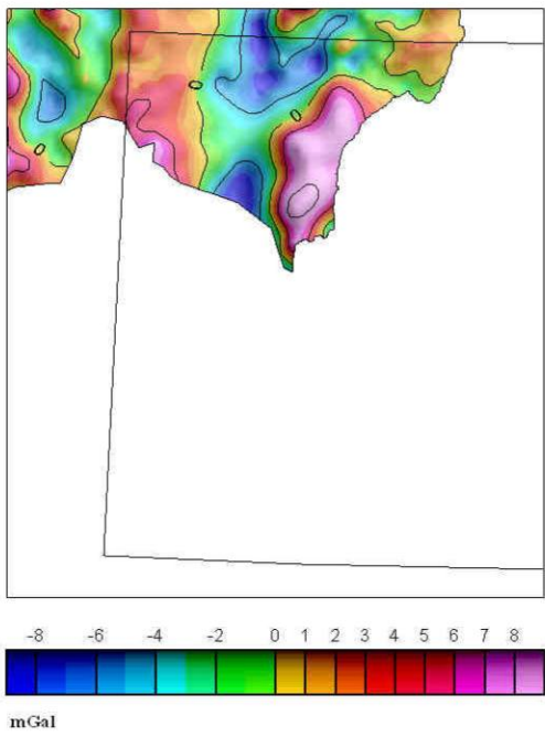
GRAVIMETRISK RESIDUALKART
