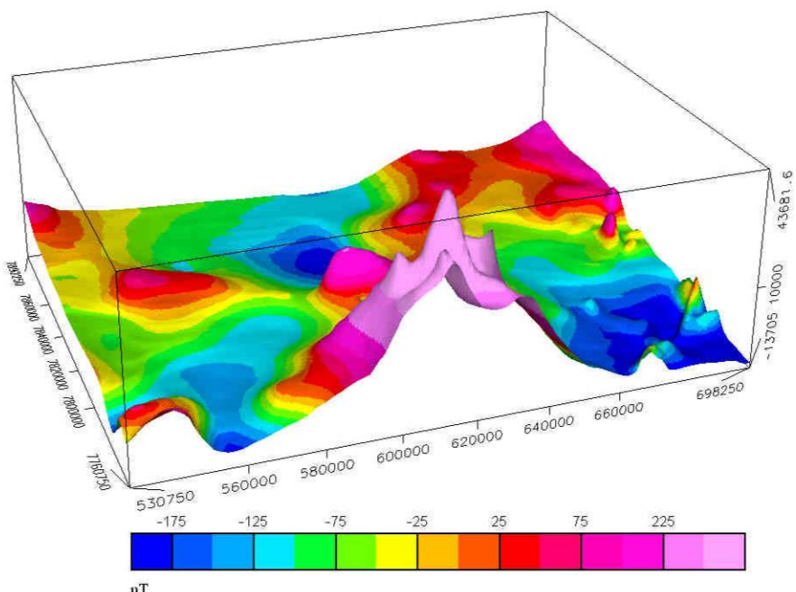
AEROMAGNETISK 3D ANOMALIKART Magnetfeltet referert til DGRF 1965.0 AEROMAGNETIC 3D ANOMALY MAP Magnetic field referred to DGRF 1965.0
