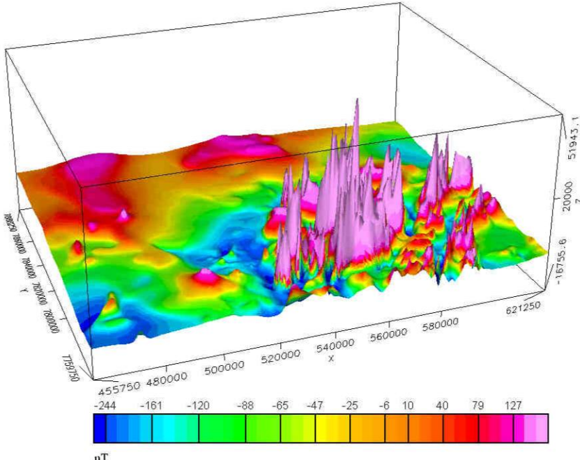
AEROMAGNETISK 3D ANOMALIKART Magnetfeltet rettet til DGRF 1965.0
