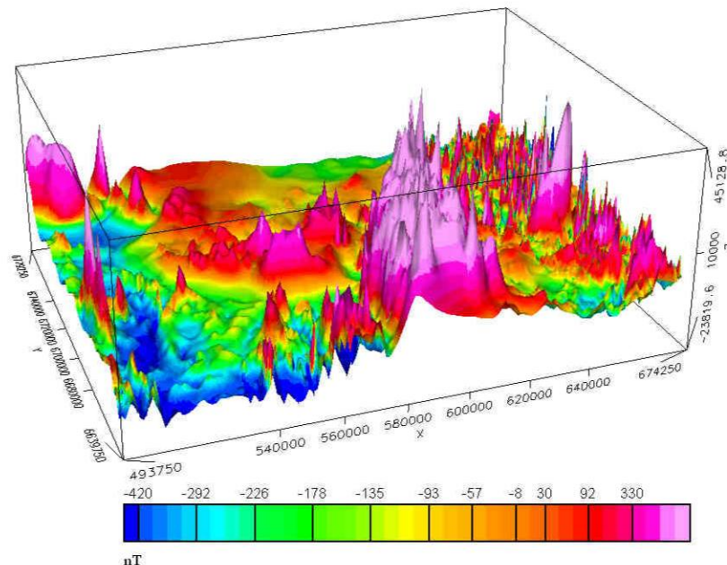
AEROMAGNETISK ID ANOMALIKART Magnetfeltet referert til DGRF 1965.0 AEROMAGNETIC ID ANOMALY MAP Magnetic field referred to DGRF 1965.0
