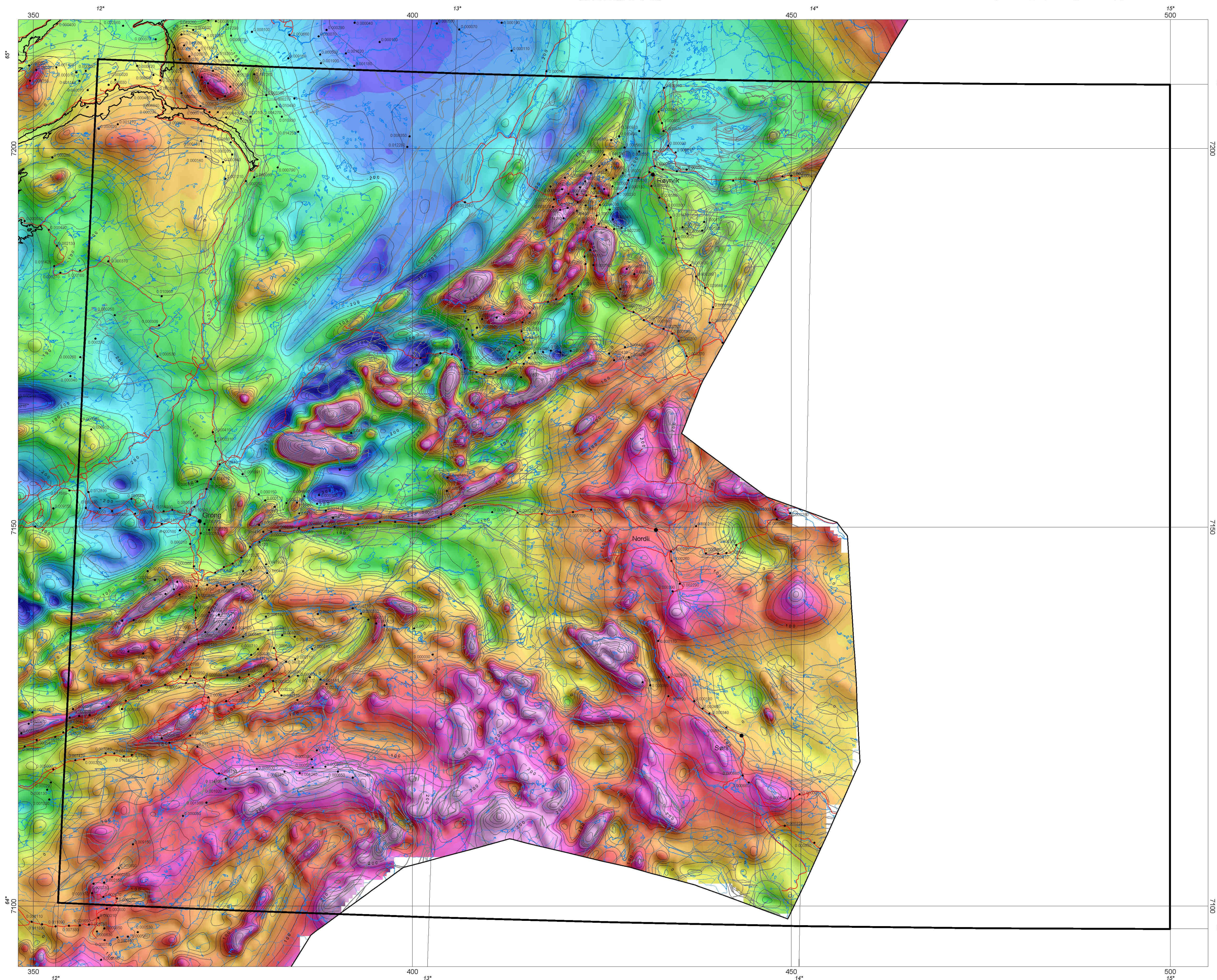
TYNGDEANOMALIKART Terrængkorrigerde bouguer anomalier GRAVITY ANOMALY MAP Terrain-corrected bouguer anomalies
