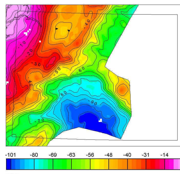
TYNGDEANOMALIKART Terrængkorrigerde bouguer anomalier GRAVITY ANOMALY MAP Terrain-corrected bouguer anomalies
