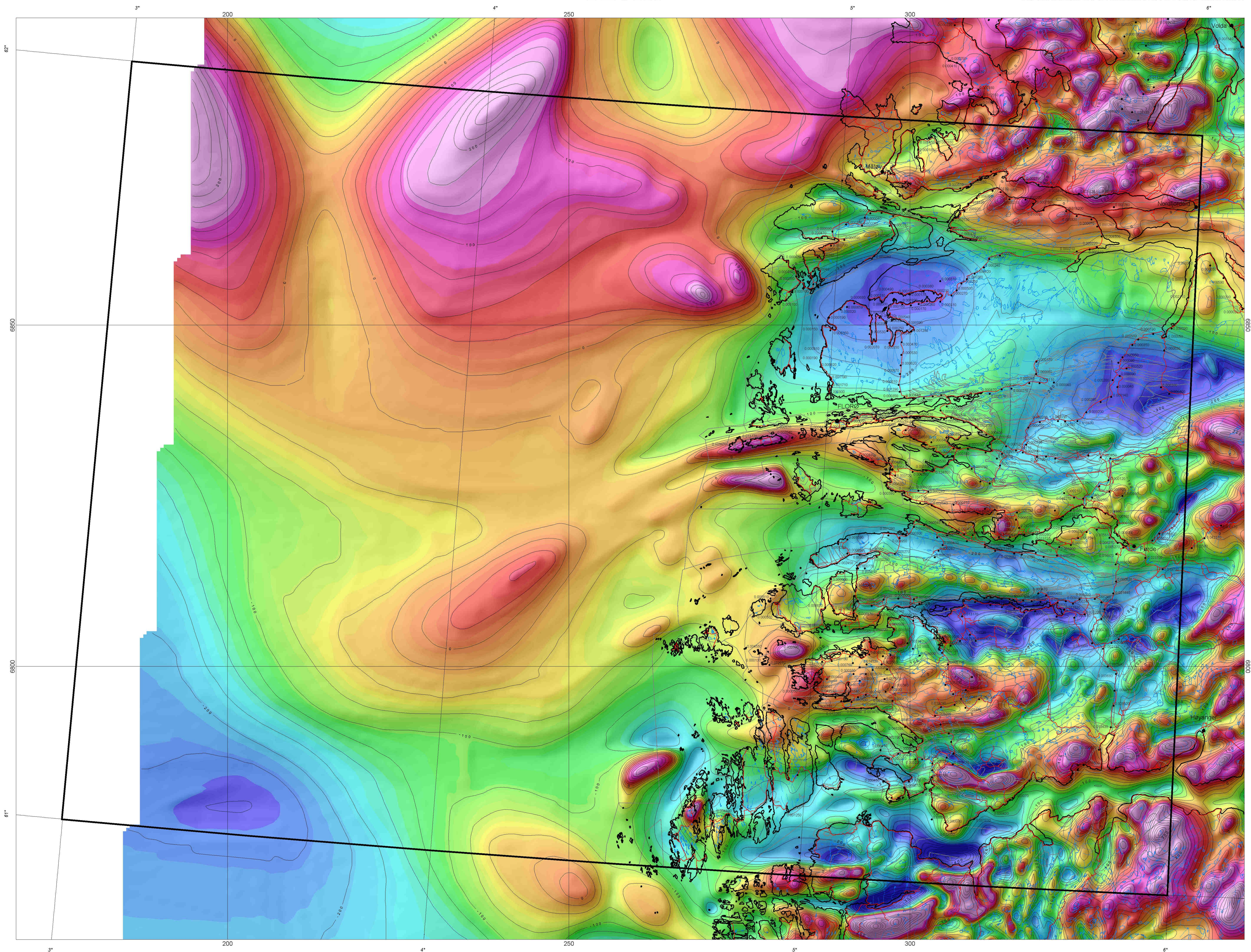
TYNGDEANOMALIKART Teterrngkorrigerte bongner anomalies
