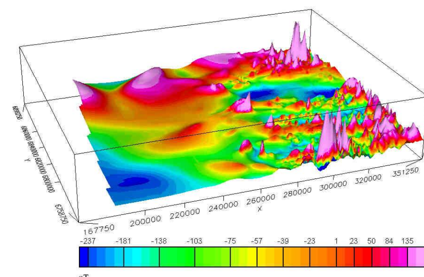
AEROMAGNETISK 3D ANOMALIKART Magnetfeltet refereret til DGRF 1965.0 AEROMAGNETIC 3D ANOMALY MAP Magnetic field referred to DGRF 1965.0
