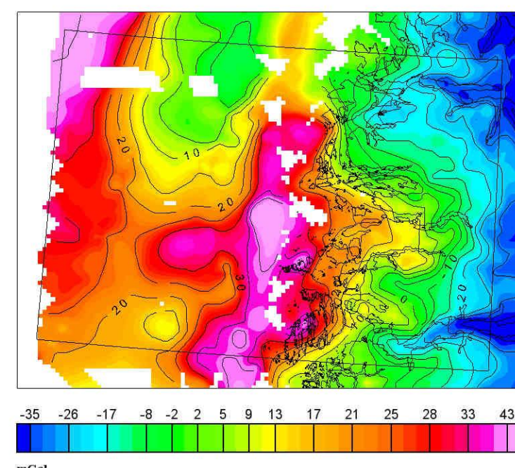
TYNGDEANOMALIKART Teterrngkorrigerte bongner anomalies
