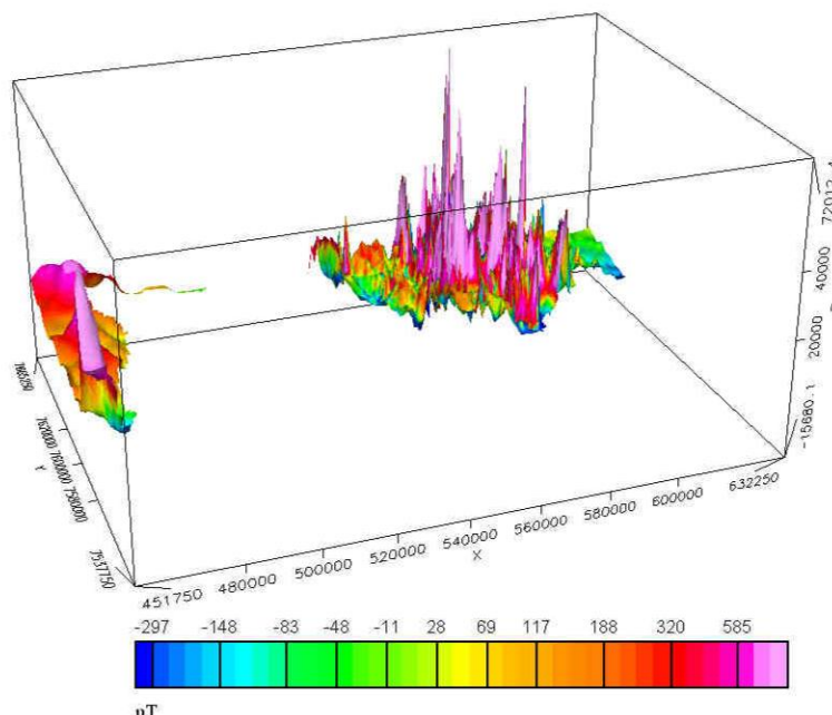
AEROMAGNETISK ANOMALIKART Magnetfeltet referert til DGRF 1965.0 AEROMAGNETIC ANOMALY MAP Magnetic field referred to DGRF 1965.0
