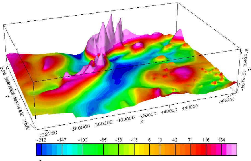
AEROMAGNETISK 3D ANOMALIKART Magnetfeltet referert til DGRF 1965.0 AEROMAGNETIC 3D ANOMALY MAP Magnetic field referred to DGRF 1965.0
