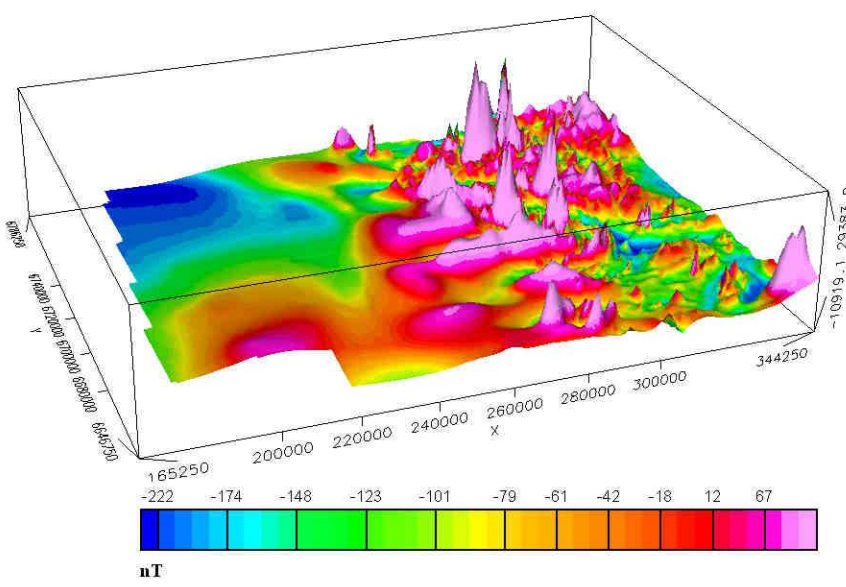
AEROMAGNETISK ANOMALIKART Magnetfeltet referert til DGRF 1965.0 AEROMAGNETIC ANOMALY MAP Magnetic field referred to DGRF 1965.0
